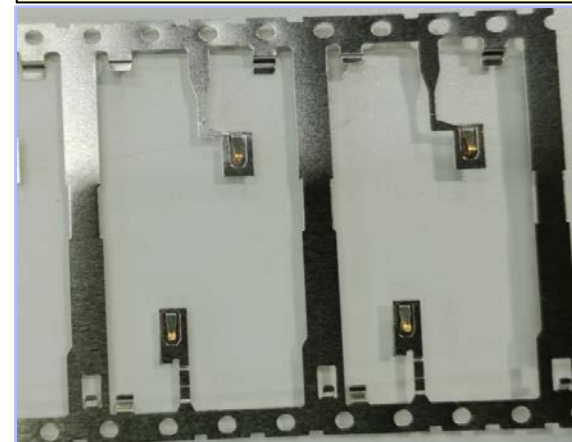
点镀----弹片
