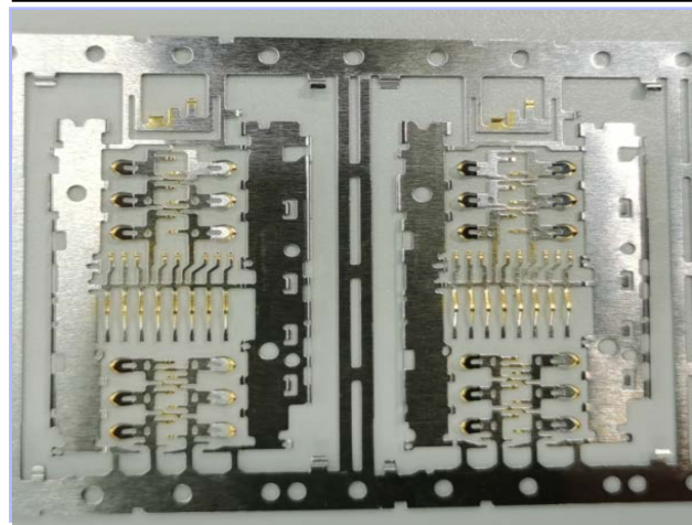
点镀----端子
