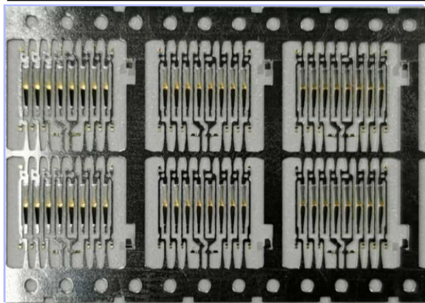
点镀----端子
